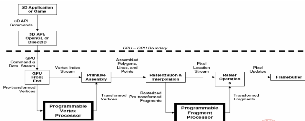
Fig. 1. GPU Pipeline
